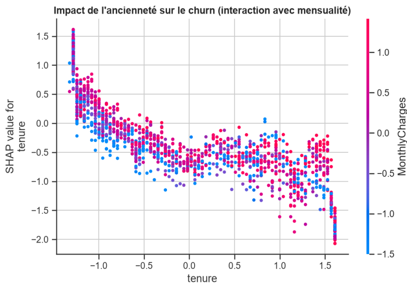
Figure 17. SHAP Dependence Plot - interaction ancienneté / mensualité.
