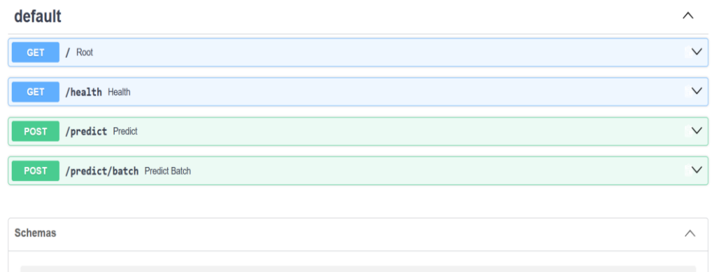
Figure 20. Documentation interactive FastAPI - 4 endpoints disponibles.
